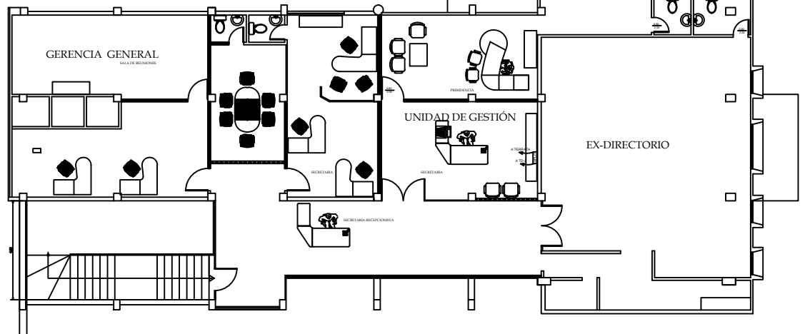
PLANTA ALTA GENERAL EXISTENTE
